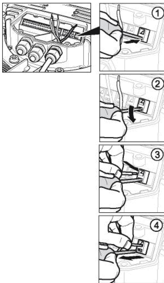
Ábra 2: Vezetékek és kapcsok csatlakoztatása
