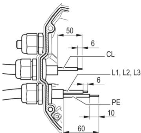
Ábra 1: Ajánlott lecsupaszítási méretek mm-ben (csatlakozódobozban) Jelmagyarázat: CL= Vezérlőkábelek
