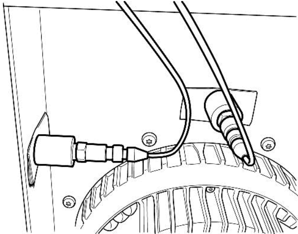
Ábra 3: A rezgésmérés példaszerű ábrázolása. Az érzékelők elrendezése az adott készüléktől és a beépítési helyzettől függ.
